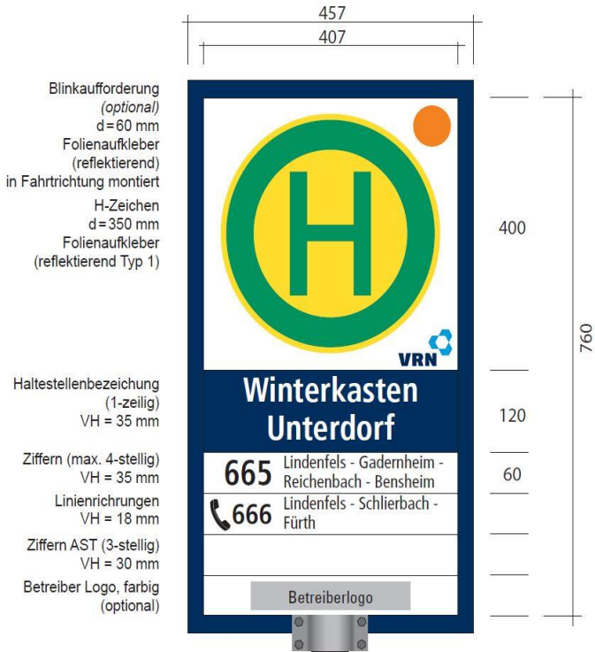
Abb. 32: Wechselschildsystem Variante 1
